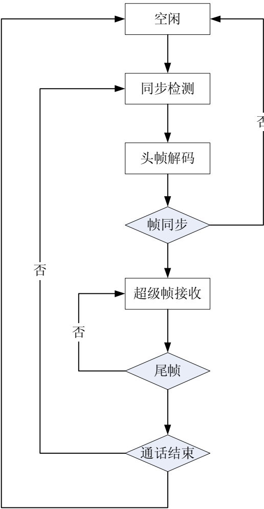
图 B.4 接收处理流程
