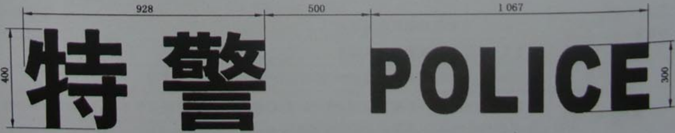
图 5 公安特警专用车辆车身两侧中英文组合规格和主要尺寸(方式三)
