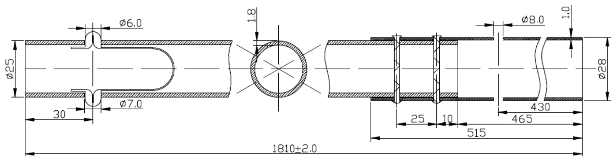
图 B.3 山墙地杆结构及主要尺寸
