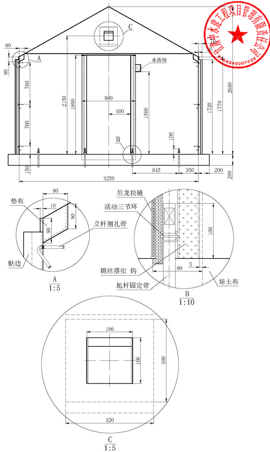
图A.3 篷体开门山墙里结构及主要尺寸
