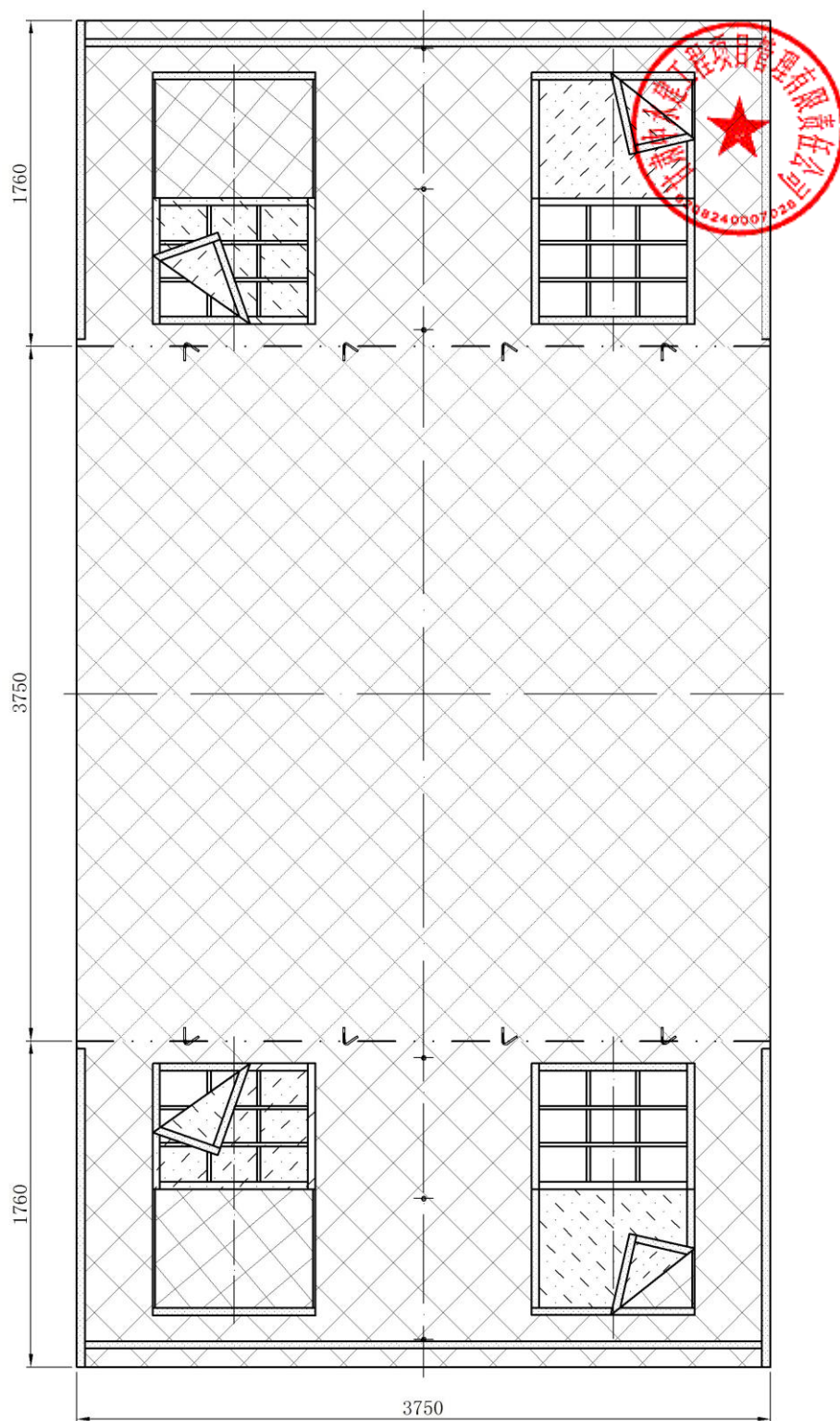
图 A. 15 棉内胆篷顶和侧墙面结构及主要尺寸
