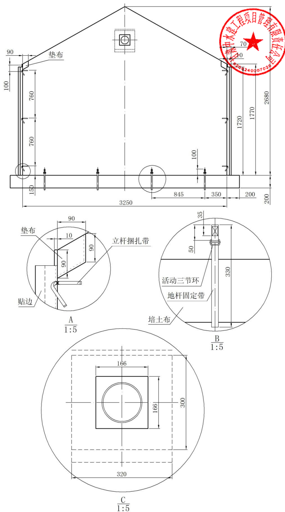
图A.5 篷体无门山墙里结构及主要尺寸
