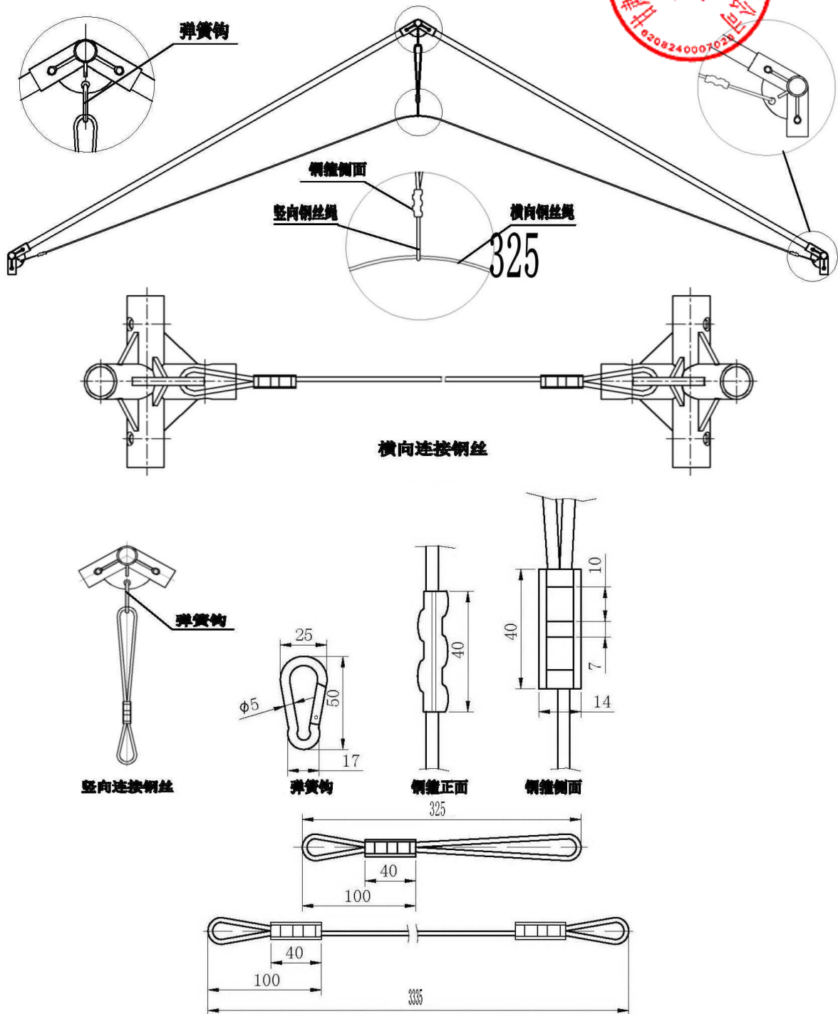
B.8 钢丝拉绳结构及主要尺寸
