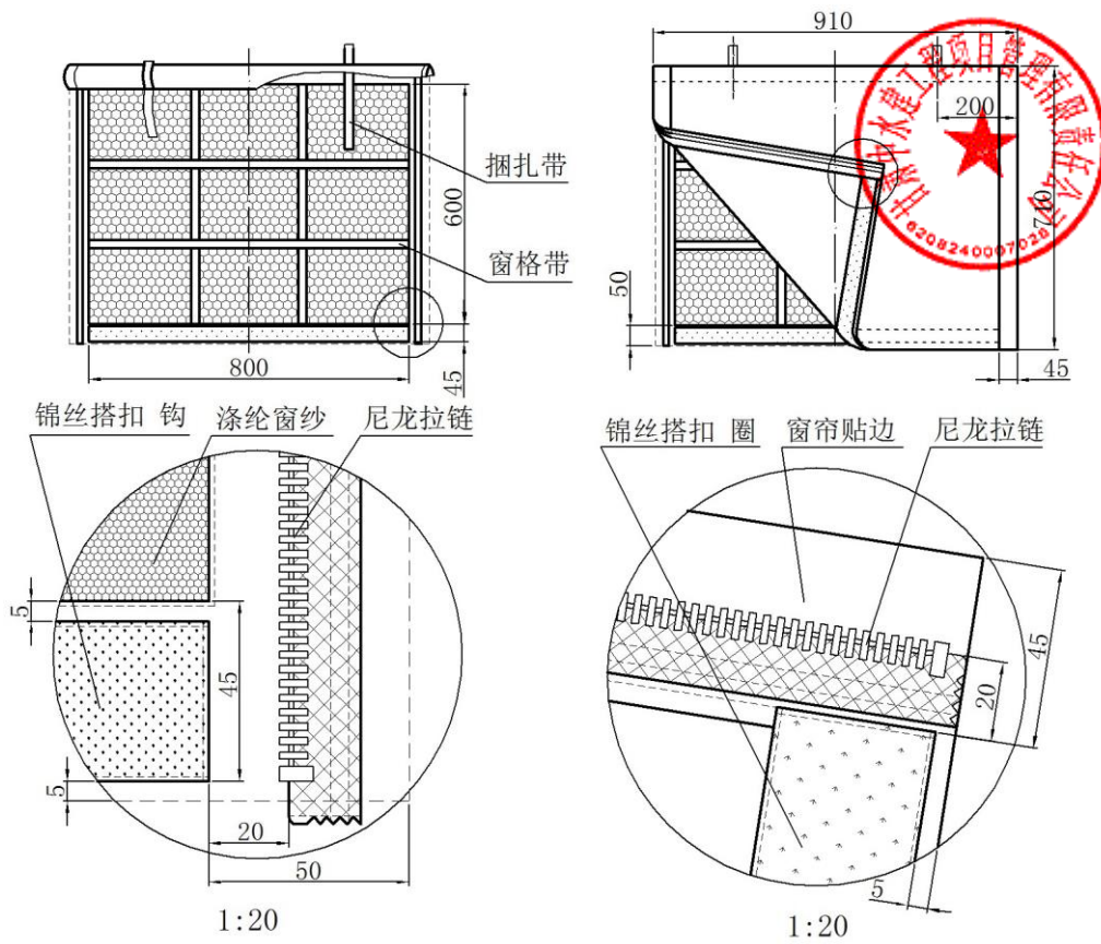
图A.9 篷体窗帘结构及主要尺寸
