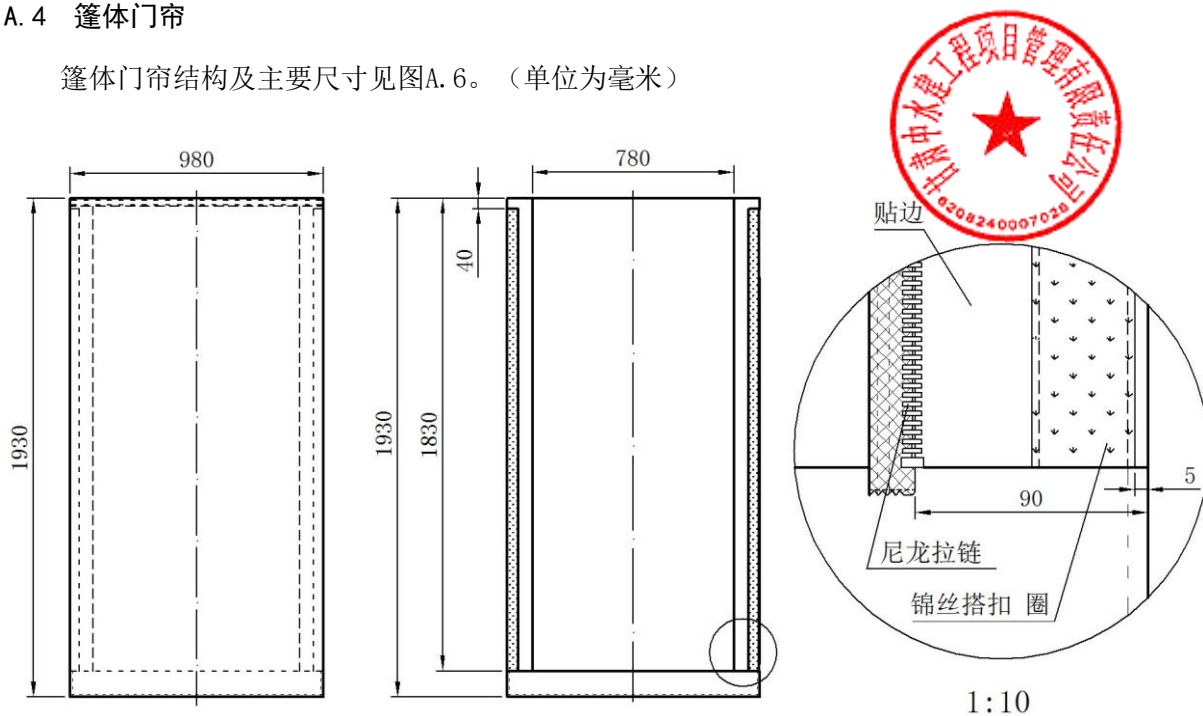
图A. 6 单篷体门帘结构及主要尺寸
