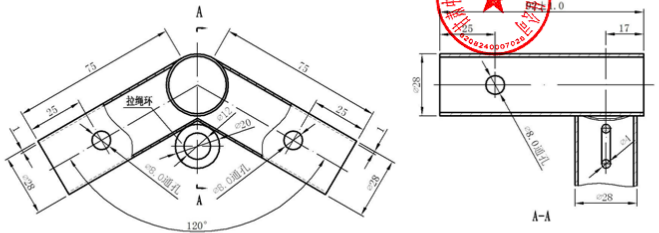
图 B.4 端架三通结构及主要尺寸
