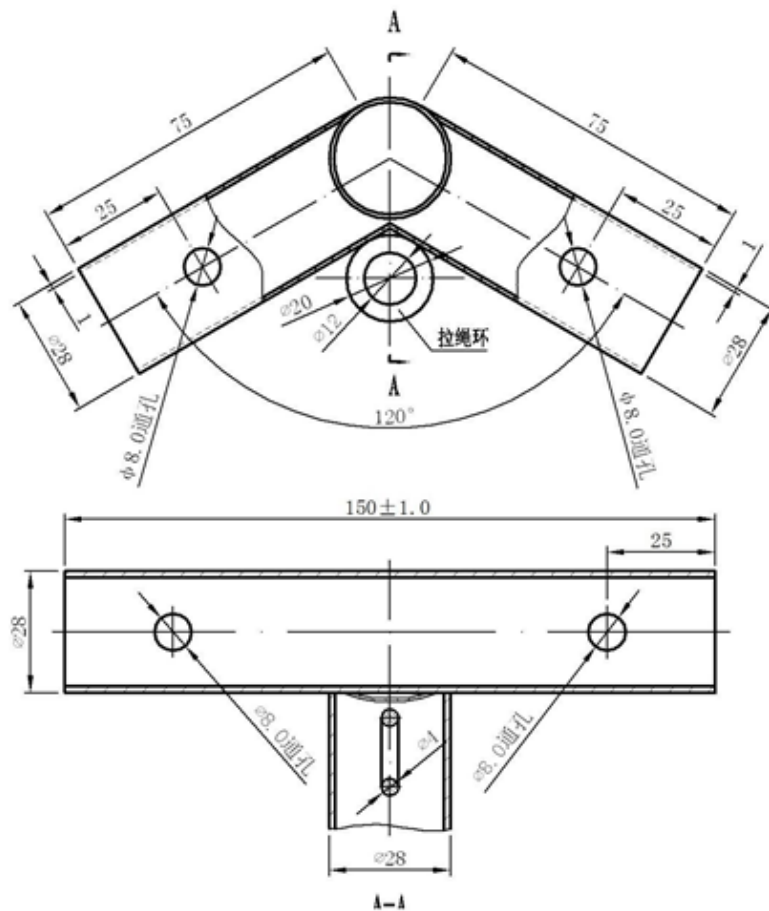
图 B.5 中架四通结构及主要尺寸
