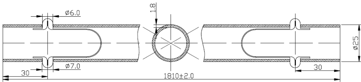
图 B.1 通用杆结构及主要尺寸
