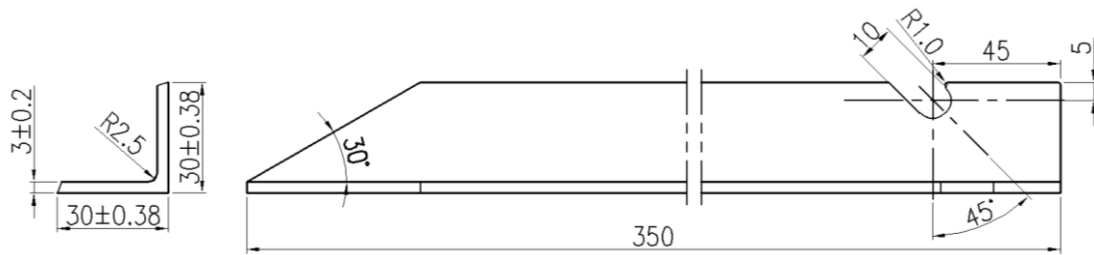
图 C.1 三角桩结构及主要尺寸
