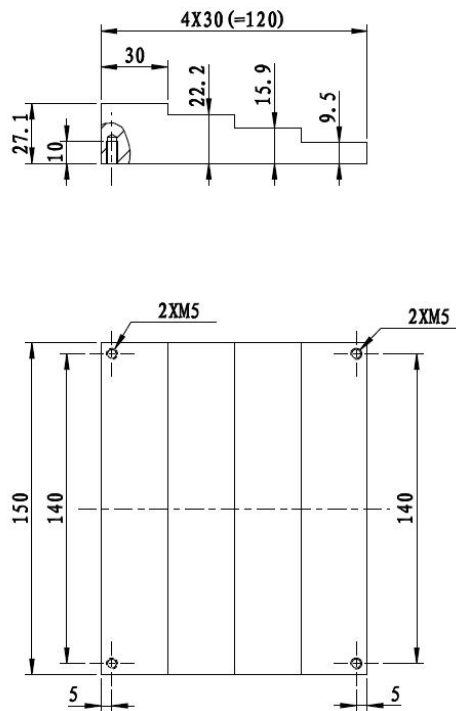
图 A. 14 测试卡 2 合金铝阶梯
