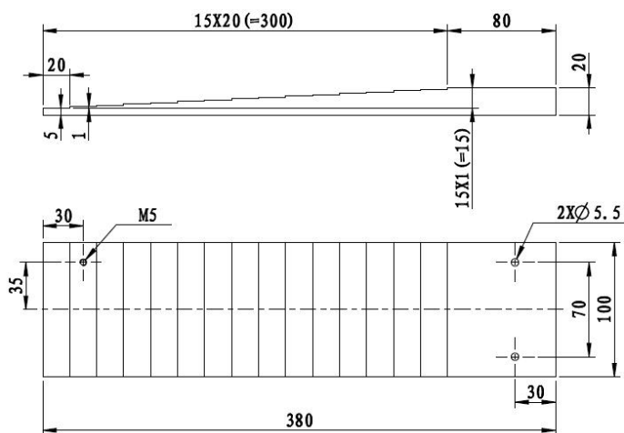
图 A. 19 测试卡 5 薄合金铝阶梯
