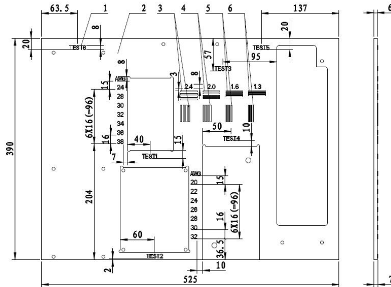
图 A.5 测试体 B 测试卡装配图
