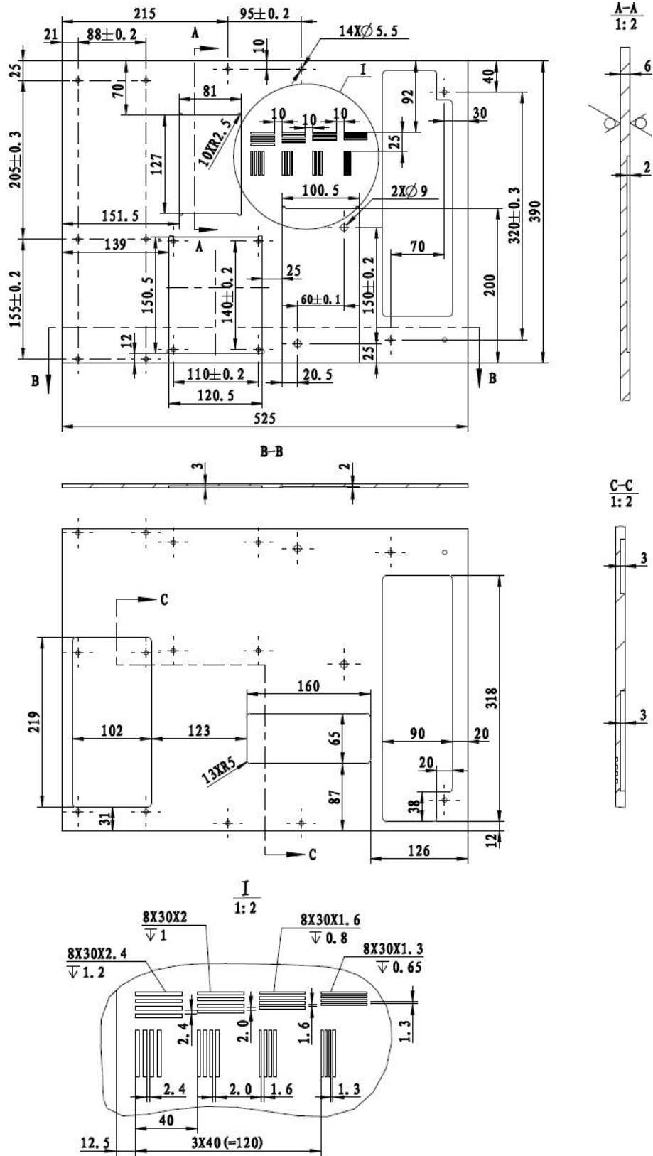
图 A.7 测试体 B 测试卡固定板
