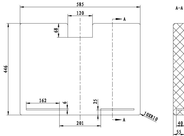
图 A.9 测试体 B 下防护衬板
