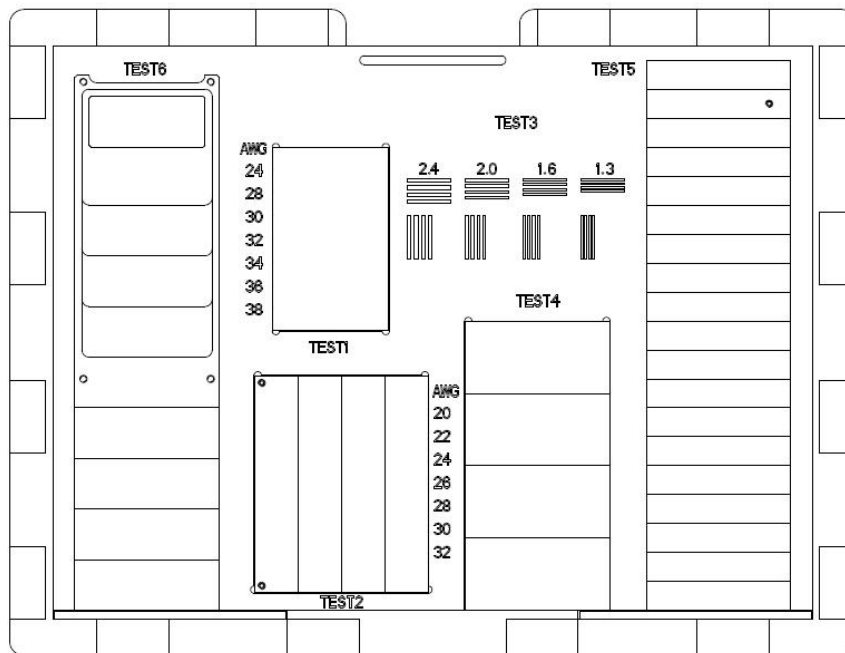
图 A.4 测试体 B 内部结构
