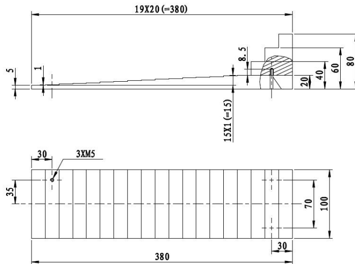
图 A. 18 测试卡 5
