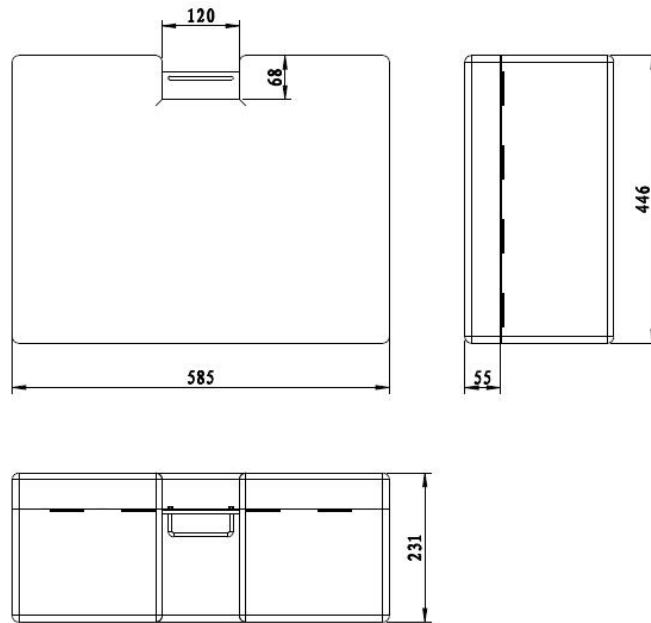
图 A.3 测试体 B 外形图
