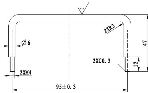
图 A.10 测试体 B 提手
