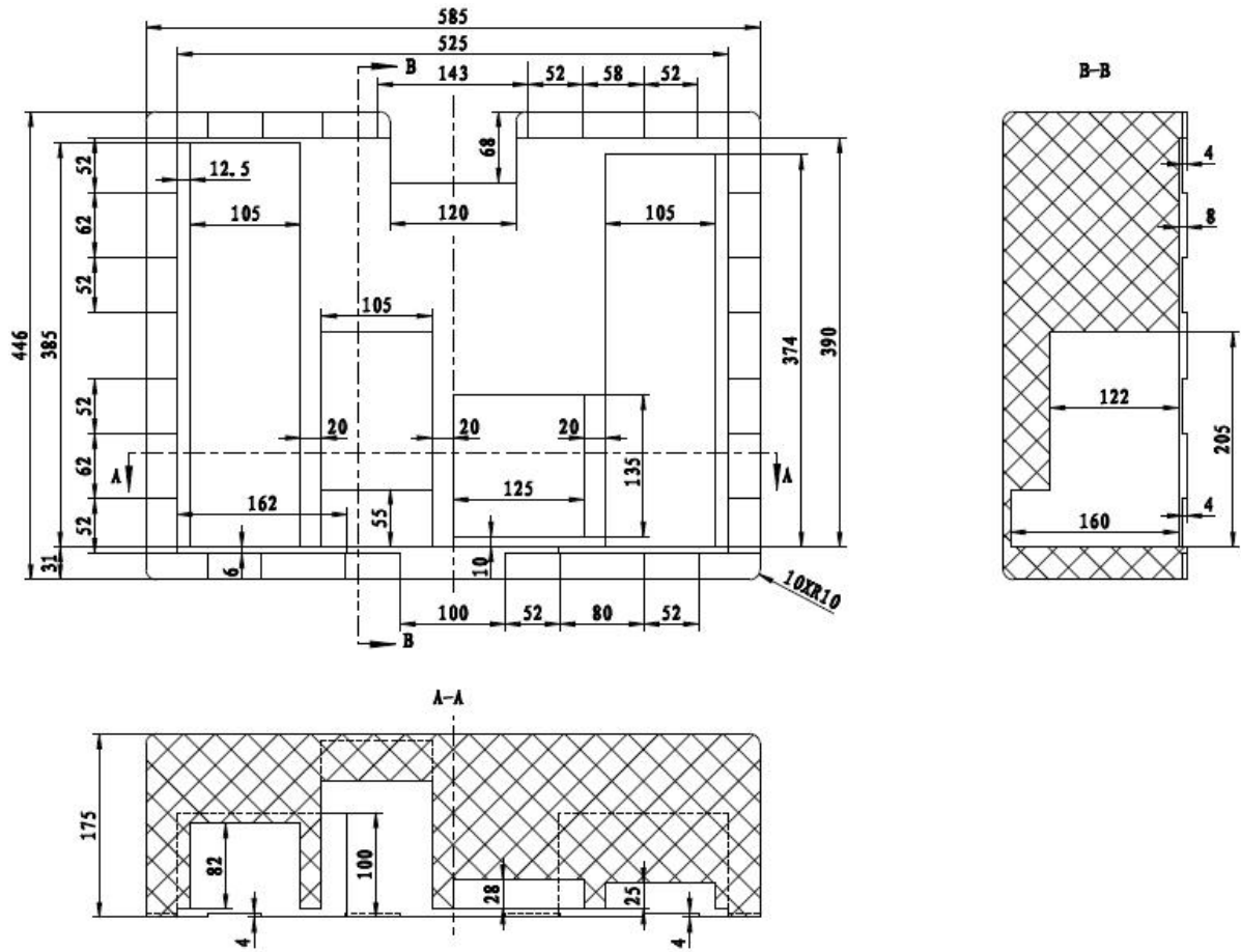
图 A.8 测试体 B 上防护衬板
