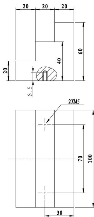
图 A. 20 测试卡 5 厚合金铝阶梯
