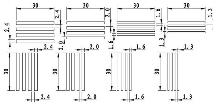
图 A.15 测试卡3尺寸图
