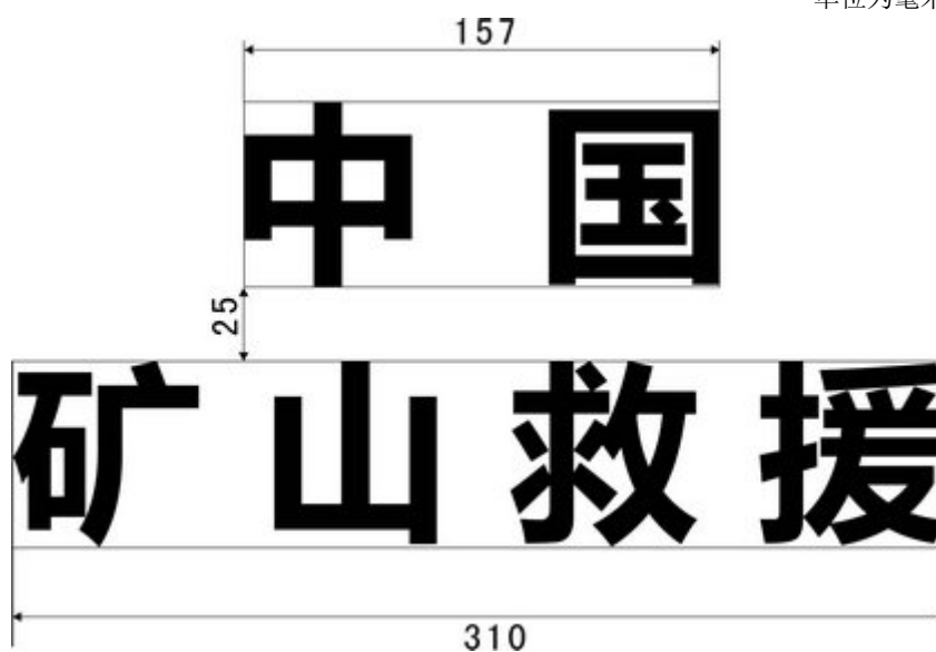
图 A.2 背部标识示意图
